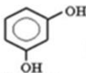
Резорцин (1,3-дигидрокси-бензол)
